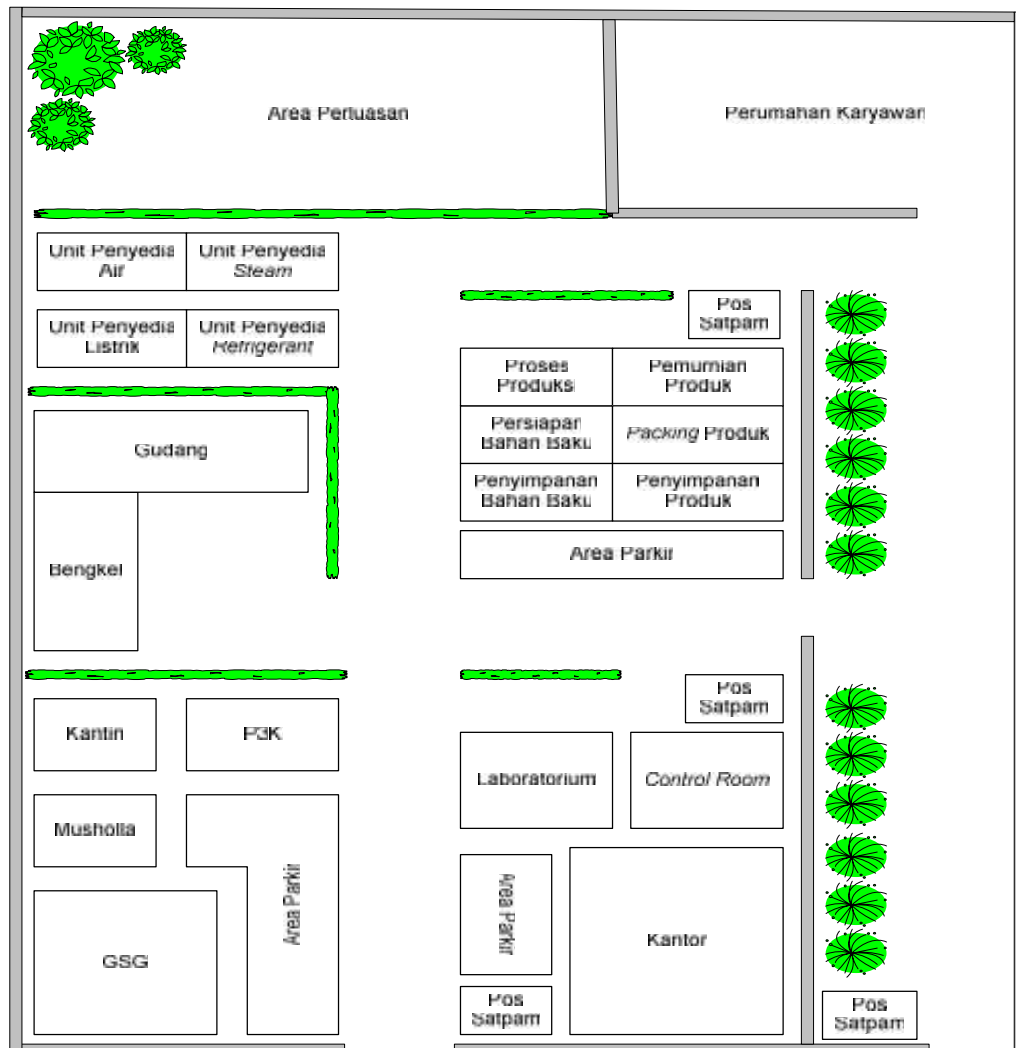
Gambar 7.1 Tata Letak Pabrik
