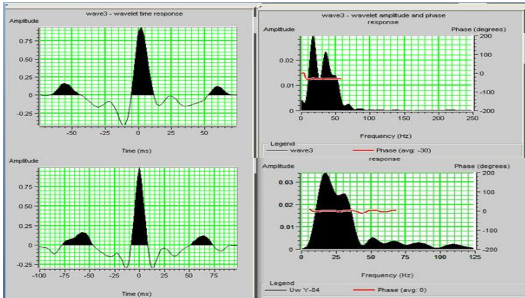
Lampiran 10 : Wavelet menggunakan sumur PRB-26 (atas) dan wavelet statistical sekitar marker (bawah)
