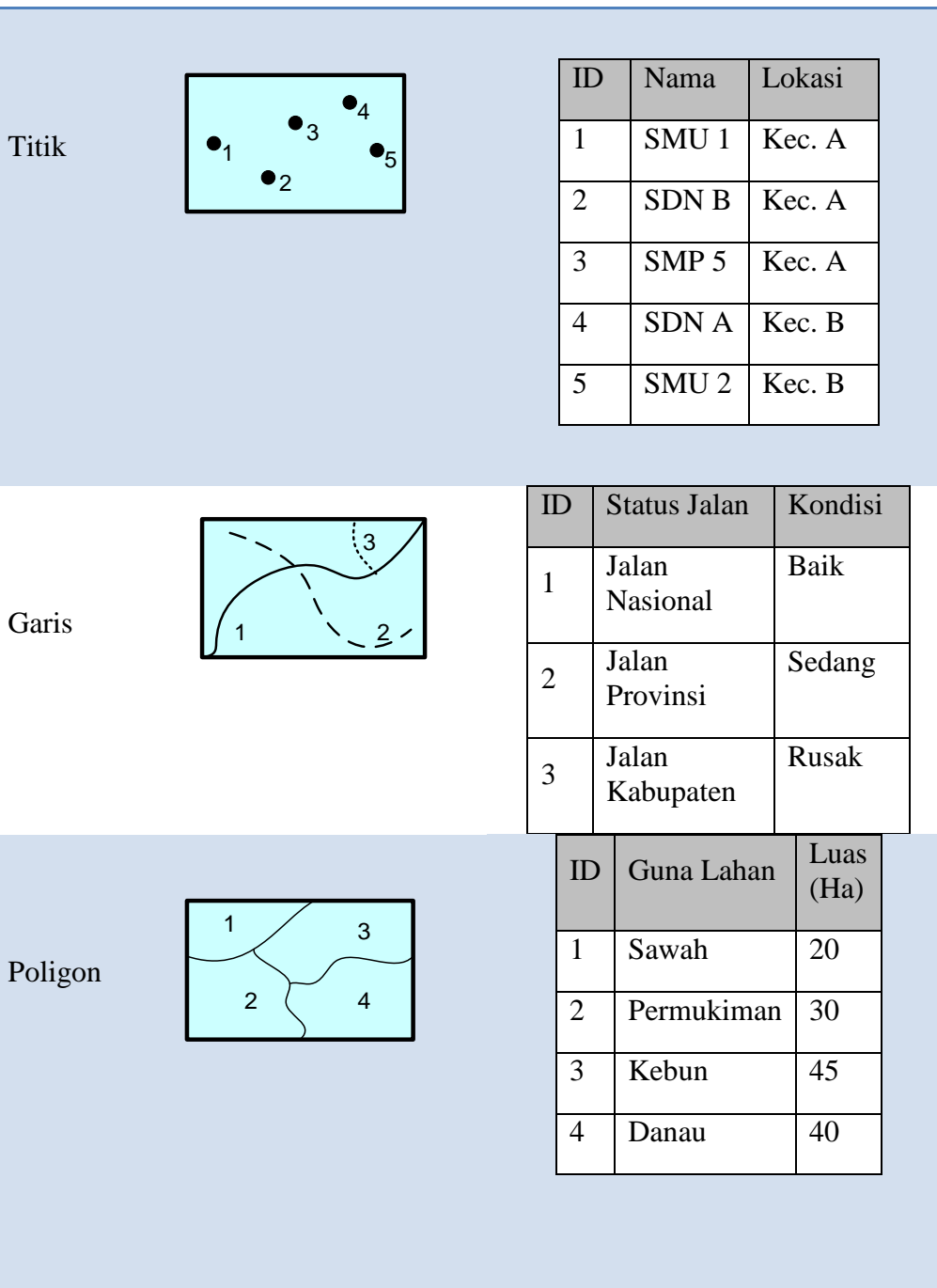
Gambar 2.3 Representasi Data Vektor dan Atributnya
