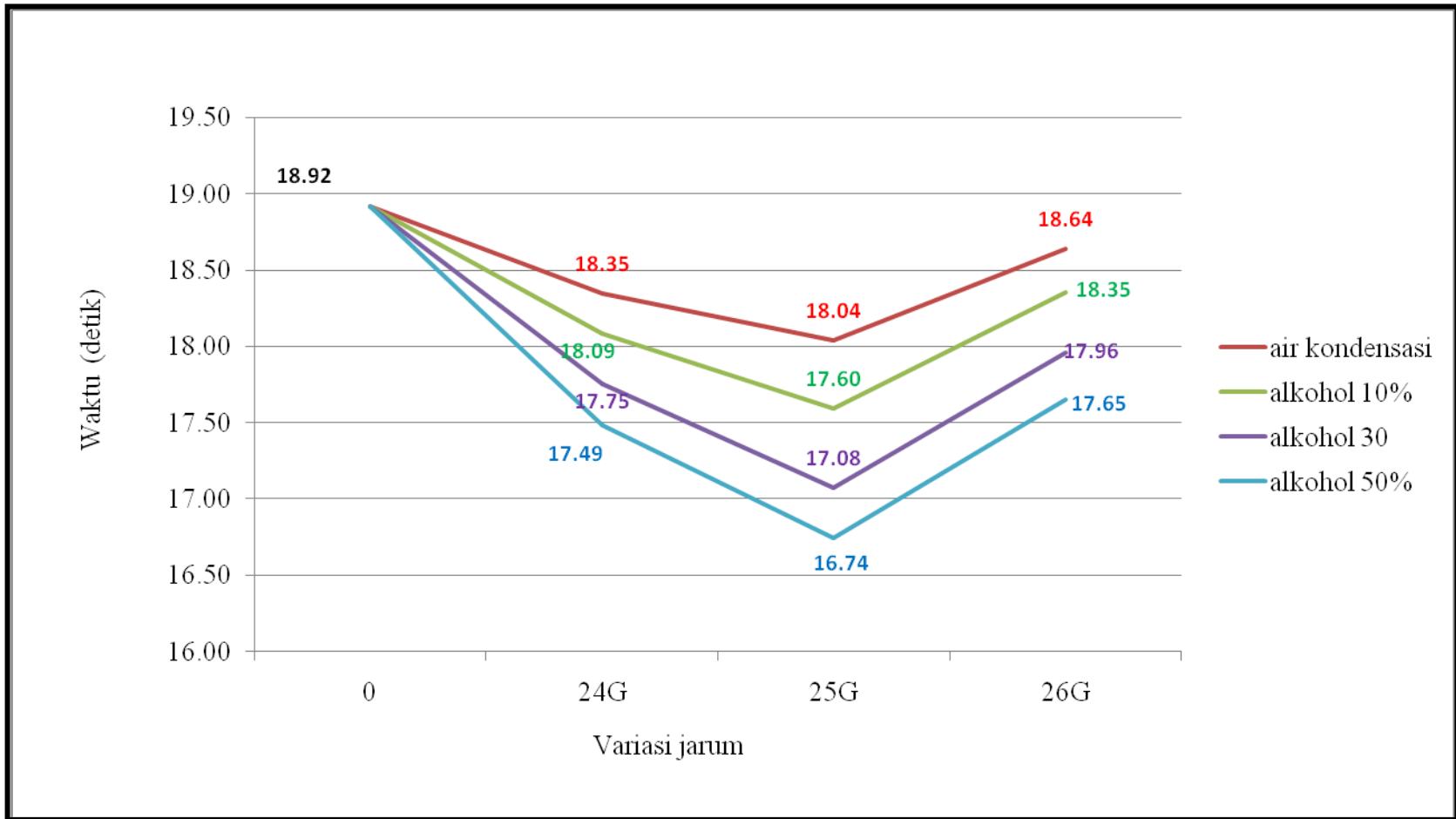
Gambar A3-3. Grafik waktu akselerasi 0-100 km/jam normal dan menggunakan Wa-i.
