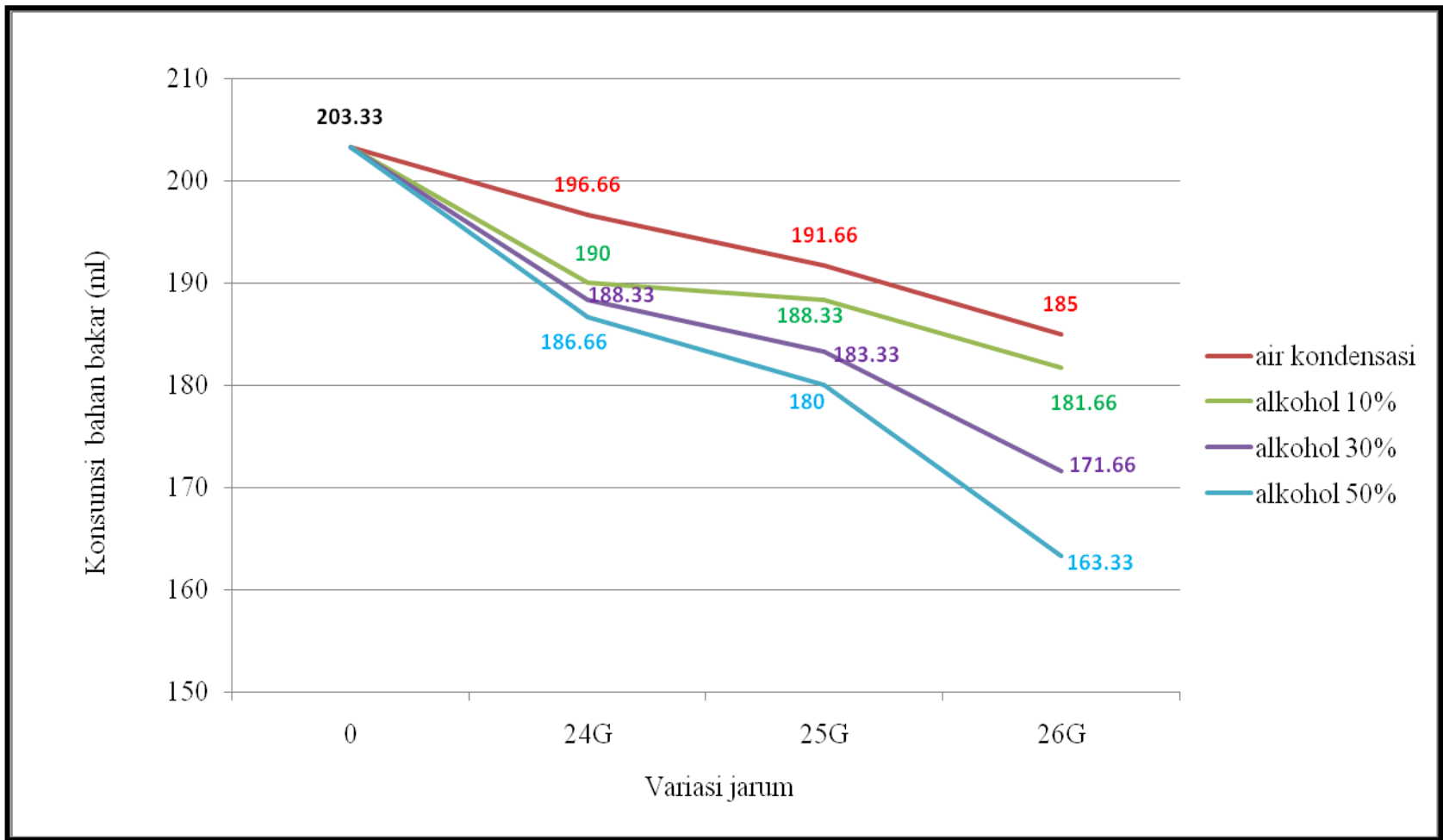
Gambar A1. Grafik konsumsi bahan bakar rata-rata pada kondisi stasioner \pm 900 rpm selama 10 menit.
