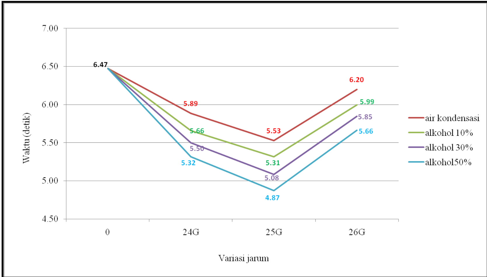
Gambar A3-1. Grafik waktu akselerasi 0-60 km/jam normal dan menggunakan Wa-i.
