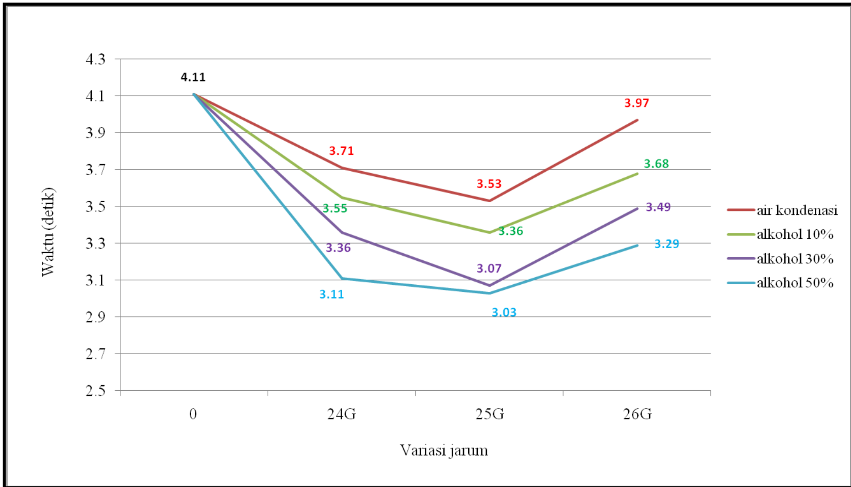
Gambar A3-2. Grafik waktu akselerasi 60-80 km/jam tanpa perpindahan persneling normal dan menggunakan Wa-i.
