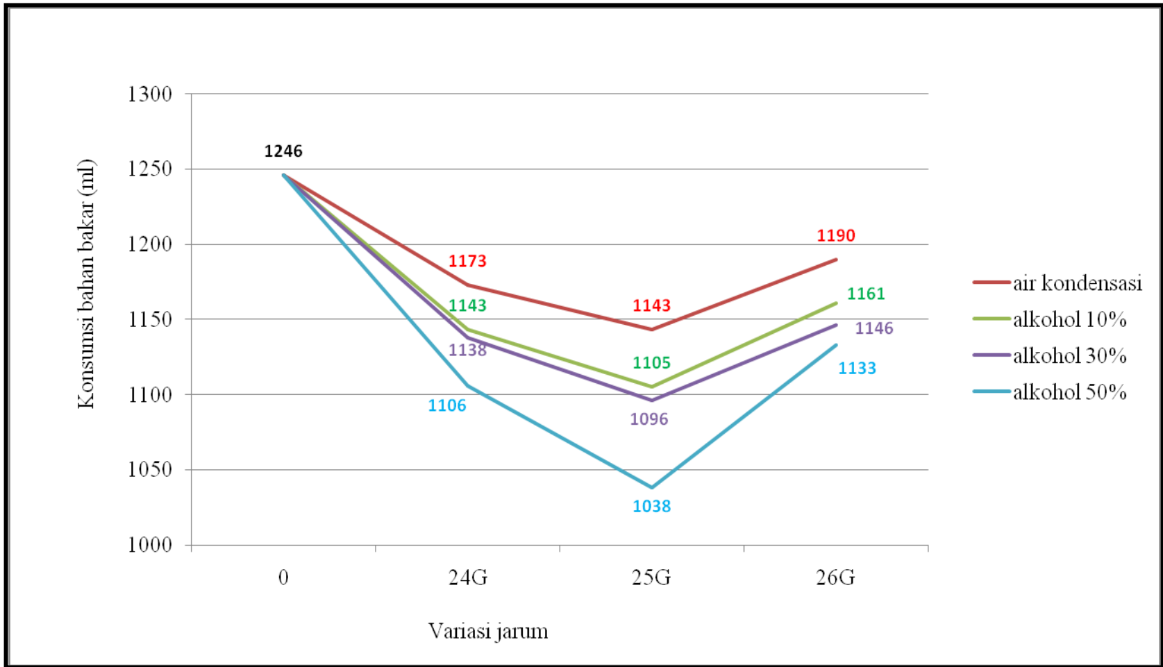
Gambar A2. Grafik konsumsi bahan bakar rata-rata pada jarak tempuh 12 km.
