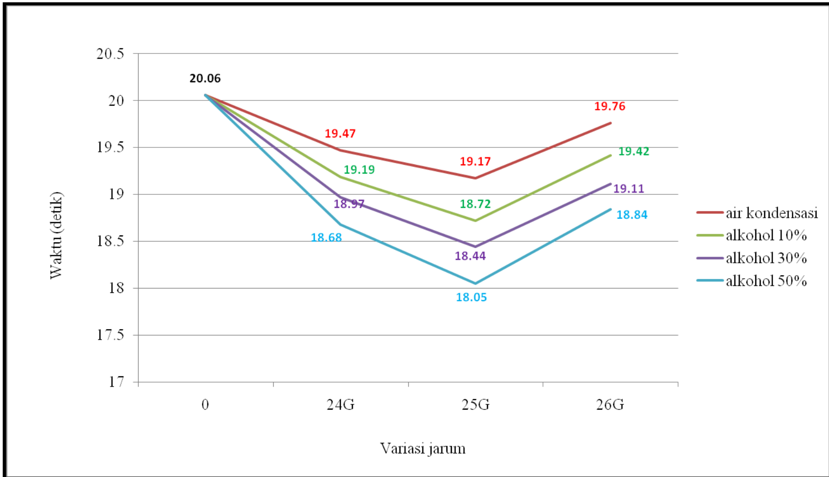
Gambar A3-4. Grafik waktu akselerasi jarak 400 m normal dan menggunakan Wa-i.
