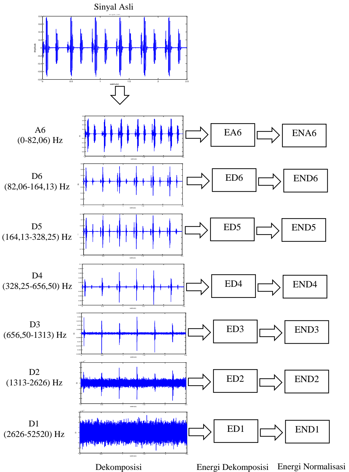
Gambar 3.7. Proses ekstraksi ciri suara jantung dengan metode energi sinyal
