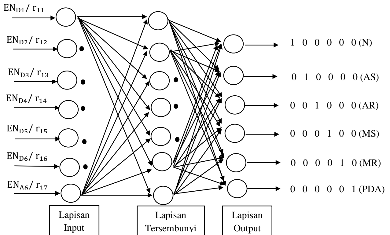
Gambar 3.8. Arsitektur jaringan syaraf tiru untuk pengenalan pola suara jantung
