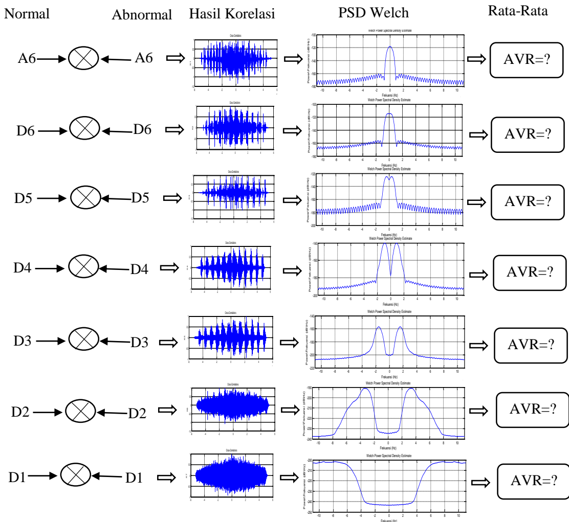
Gambar 3.6. Proses ekstraksi ciri suara jantung dengan metode dekorlet
