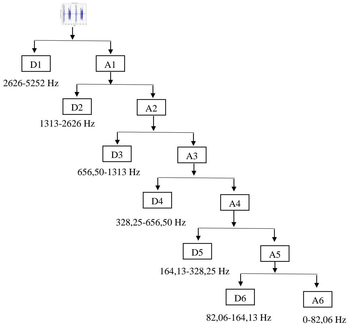
Gambar 3.5. Dekomposisi 6 tingkat sinyal suara jantung
