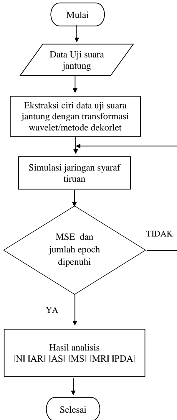
Gambar 3.11. Flowchat simulasi JST
