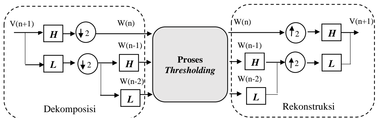
Gambar 3.4. Ilustrasi proses de-noising sinyal dengan wavelet
