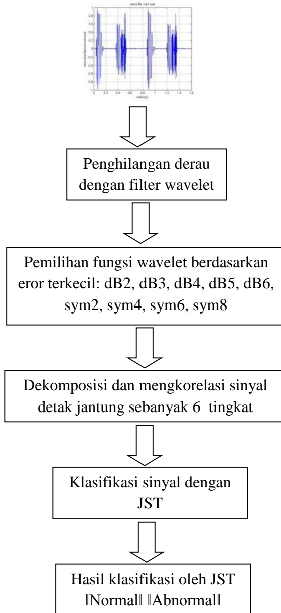
Gambar 3.9. Diagram blok pengolahan sinyal suara jantung
