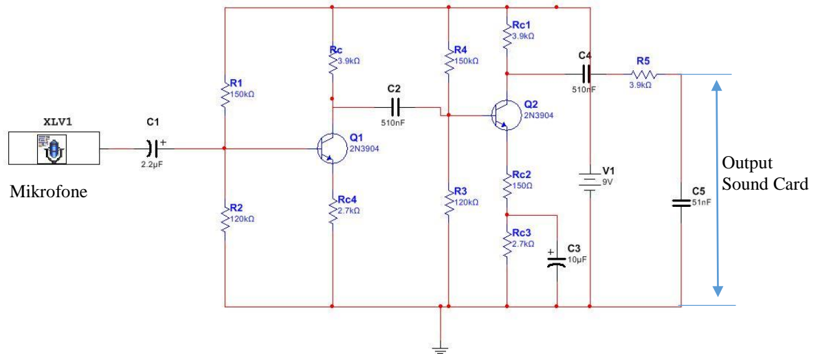
Gambar 3.2. Rangkaian penguat mikrofone dengan antarmuka sound card
