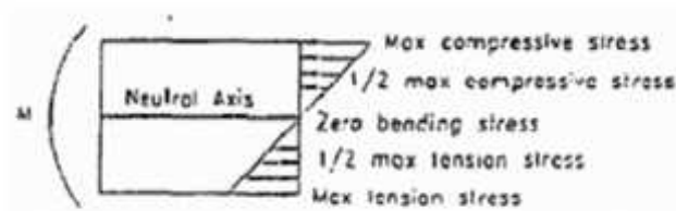
Gambar 2.4 Tegangan akibat tekuk (Maja, 2010)
