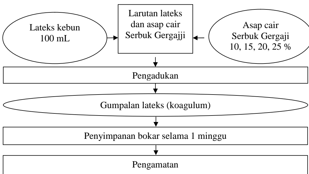
Gambar 2. Diagram alir proses koagulasi lateks dengan asap cair serbuk gergaji 5% (Asni, 2010) dimodifikasi
