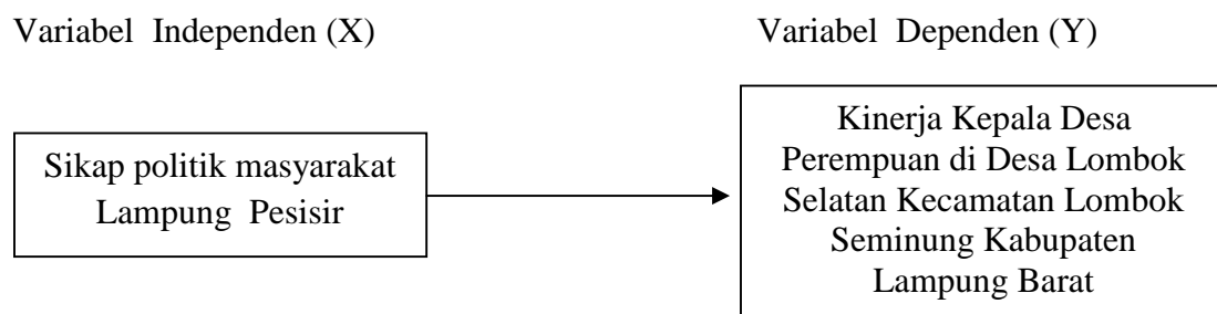
Gambar. 1 Kerangka Pikir:
