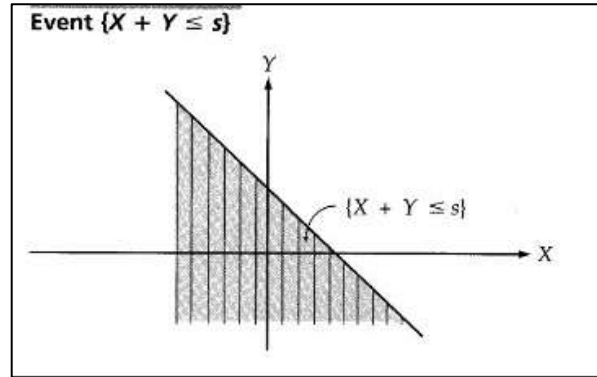
Gambar 1. Jumlah Peubah Acak S = X + Y dengan Ruang Sampel
