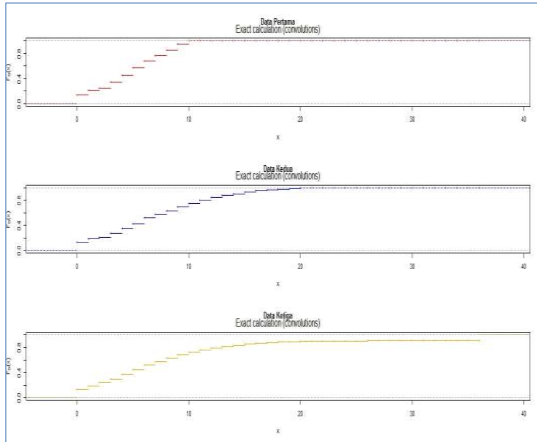
Gambar 3. Plot CDF Data Klaim Agregasi jumlah klaim berdistribusi Poisson dan besar klaim berdistribusi Rayleigh
