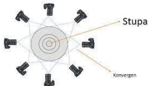
Gambar 4. Konfigurasi kamera konvergen (Amiranti, 2016)
