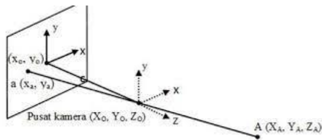
Gambar 3. Kondisi kolinear atau prinsip kesegarisan (Sumber: Atkinson, 1996)
