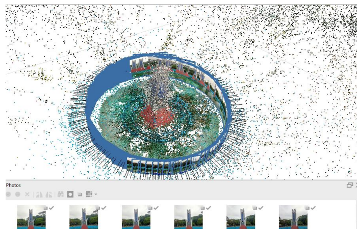
Gambar 21. Posisi kamera saat pemotretan
