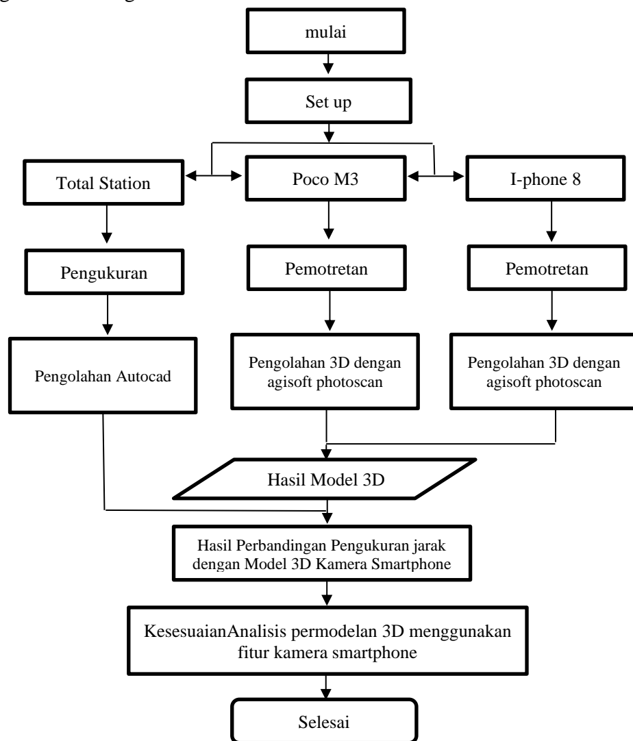
Gambar 7. Diagram Alir
