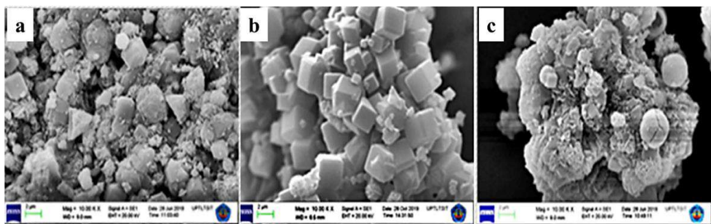
Gambar 4. Mikrograf zeolit-A dengan variasi waktu kristalisasi (a) 48 jam, (b) 72 jam, dan (c) 96 jam
