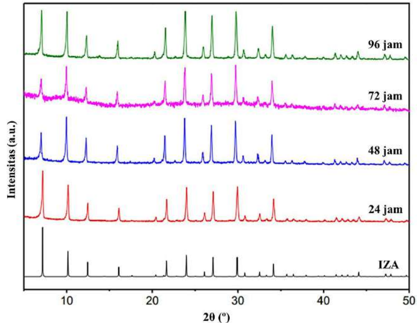
Gambar 3. Pola XRD zeolit-A hasil sintesis
