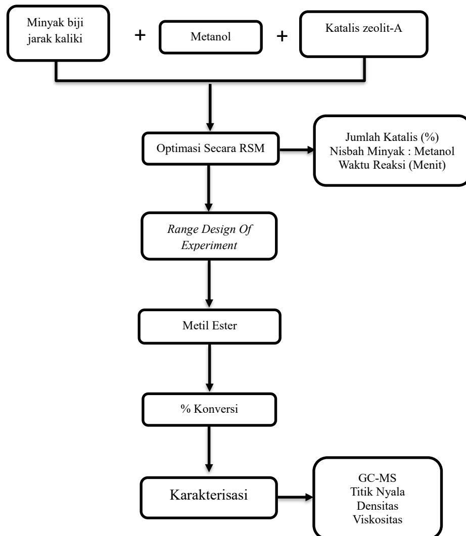
Gambar 7. Diagram alir transesterifikasi
