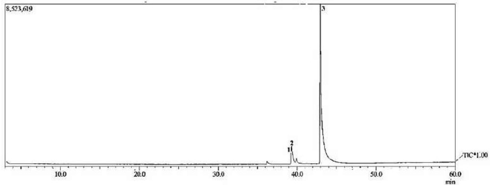
Gambar 5. Kromatogram GC-MS
