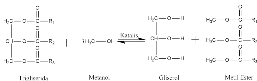
Gambar 1. Reaksi transesterifikasi
