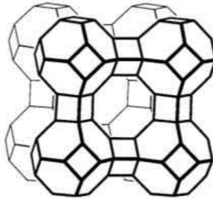
Gambar 2. Kerangka zeolit-A
