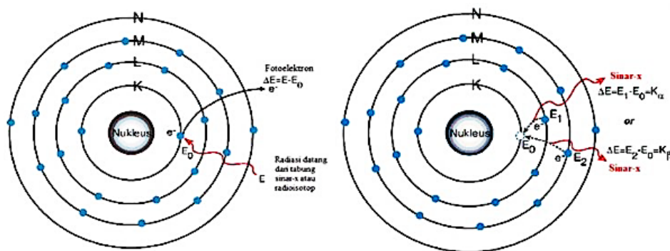
Gambar 2.1 Prinsip kerja XRF (Kalnicky & Singhvi, 2001).
