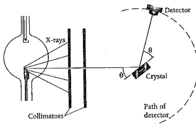
Gambar 2.2 Skema difraksi sinar-X (Cullity, 1978).
