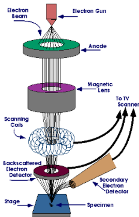
Gambar 2.4 Skema SEM (Mhadhbi, 2022).
