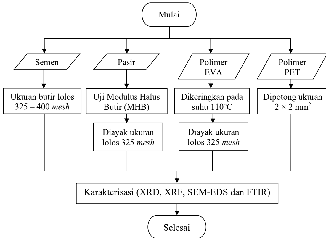
Gambar 3.1 Diagram alir preparasi dan karakterisasi bahan.
